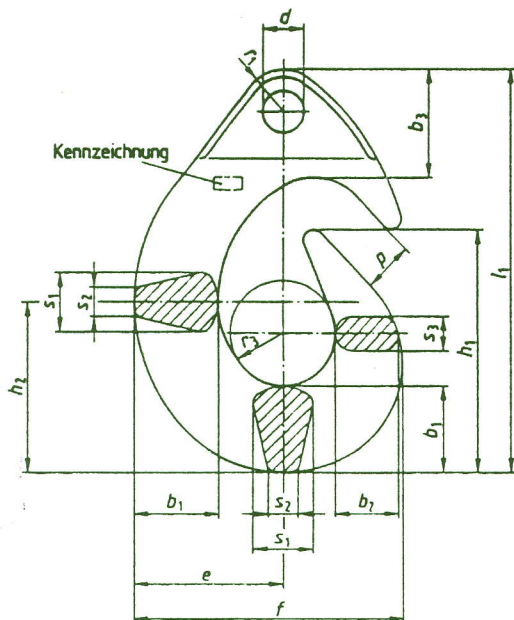
Specialkrok för maritimt bruk. (Cargo hook)
