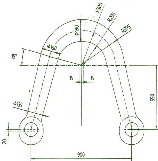
Lyftbyglar för offshore & oil drilling
